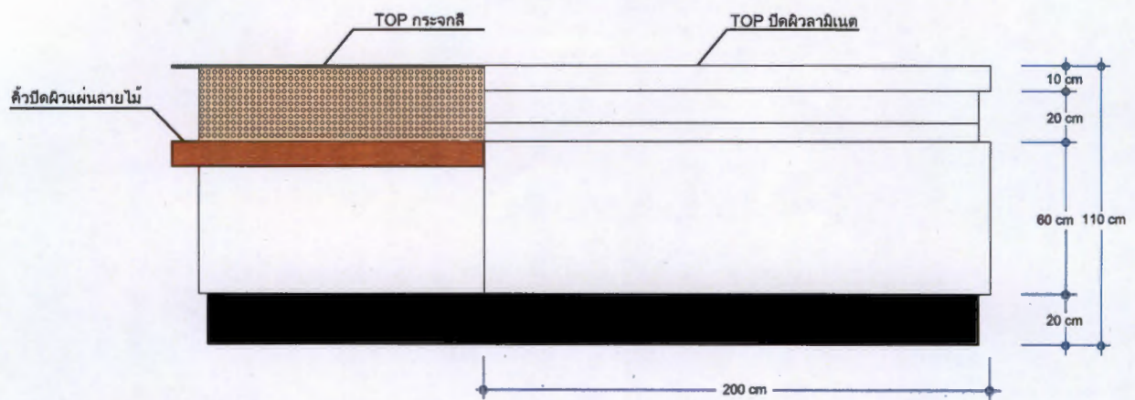
รูปด้านหน้าตัวต่อ B
