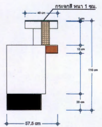
รูปด้านข้าง C
