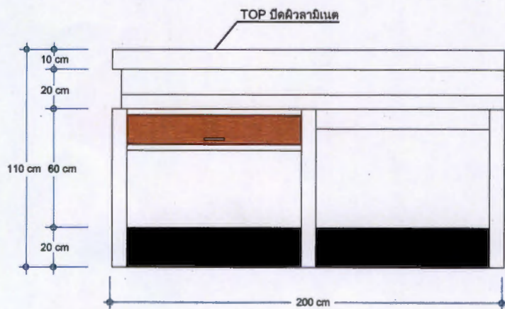
รูปด้านลิ้นชัก B
