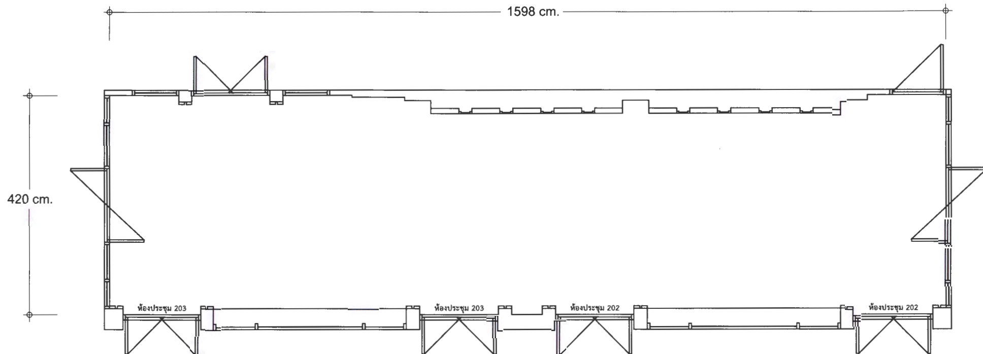
รูปแปลนด้านหน้าห้องประชุม
