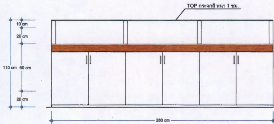
รูปด้านลิ้นชัก C
